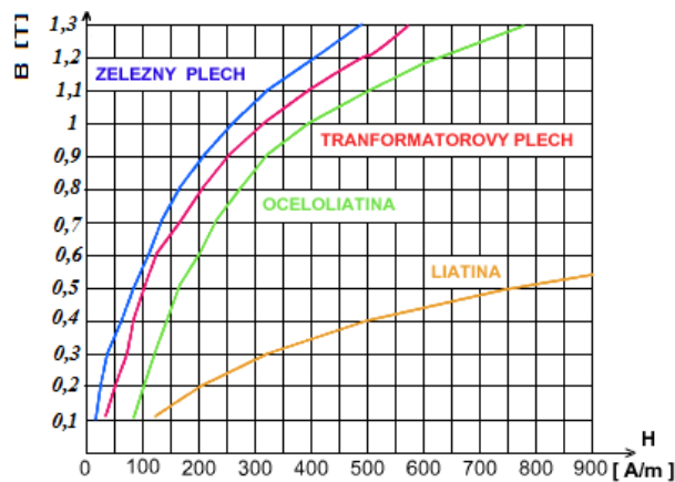
Graf 1 Magnetizačná charakteristika
